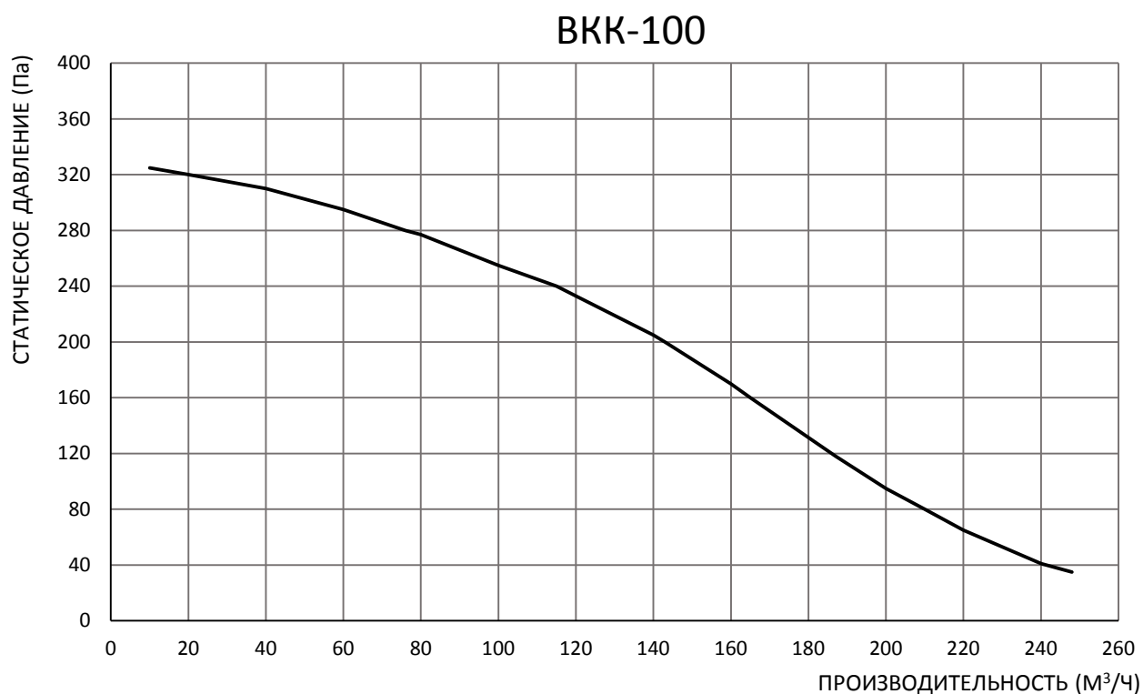
Рисунок 3. Аэродинамические характеристики ВКК.
