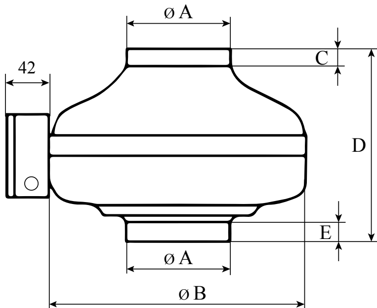
Рисунок 2. Габаритные и присоединительные размеры.
